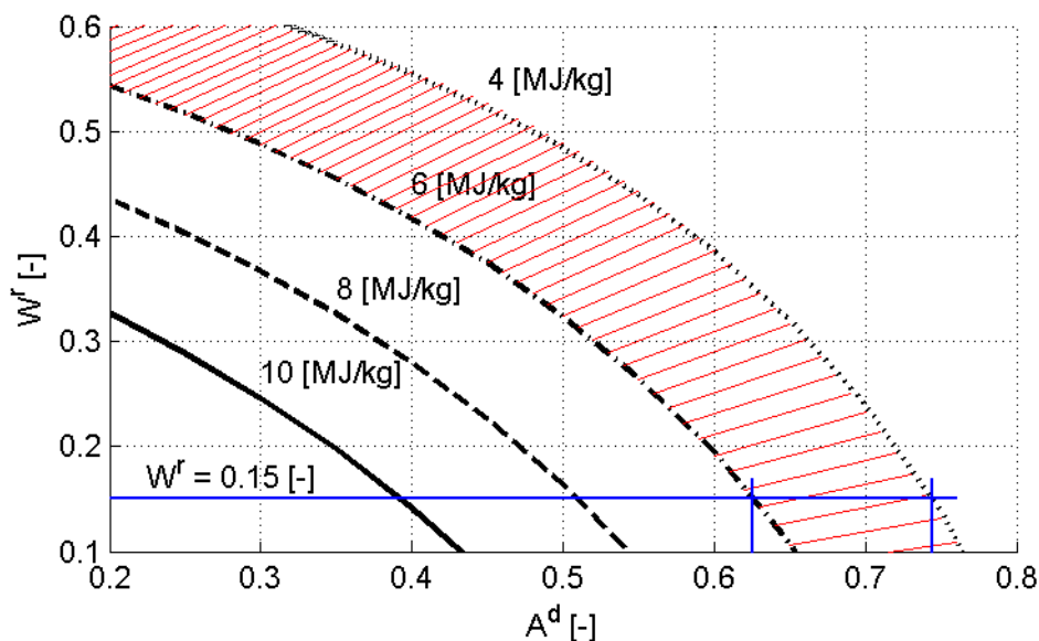
obr. 2 Diagram výhřevnosti
