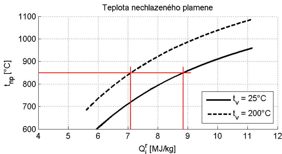
obr. 4 vliv přehřevu vzduchu na teplotu nechlazeného plamene pro A^d = 40 \%
